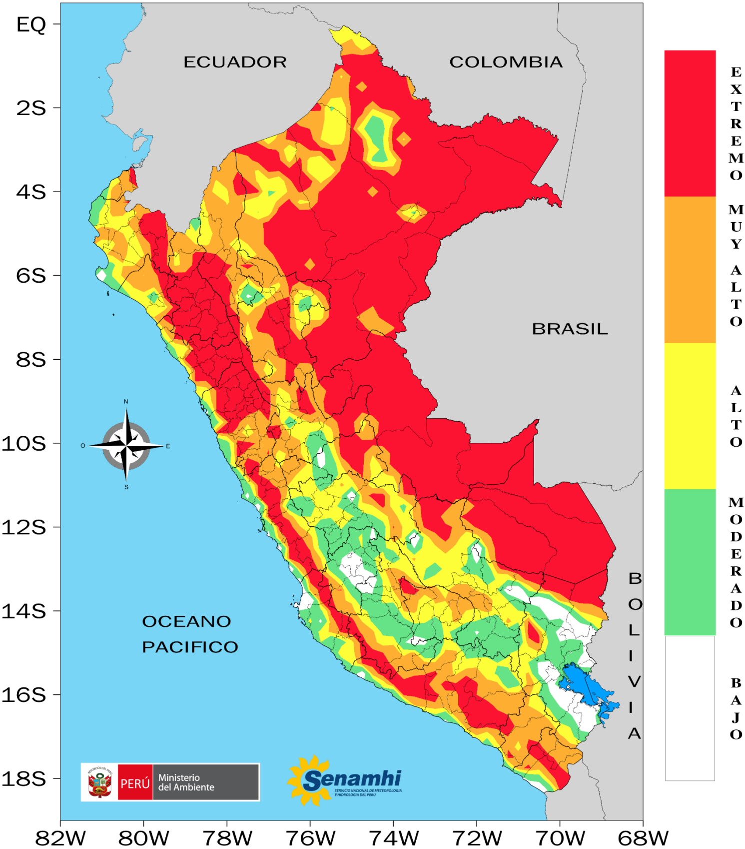
INDICE METEOROLOGICO DE INCENDIOS (FWI) 17SEP2024
